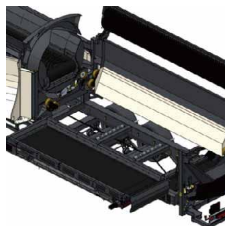
ボルト数本で容易に取り外せ メンテナンス可能なコンベアー
