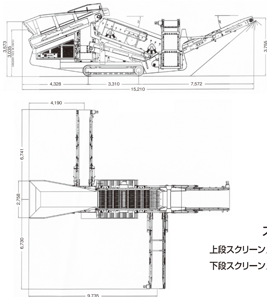
R155 寸法図 (単位: mm)
